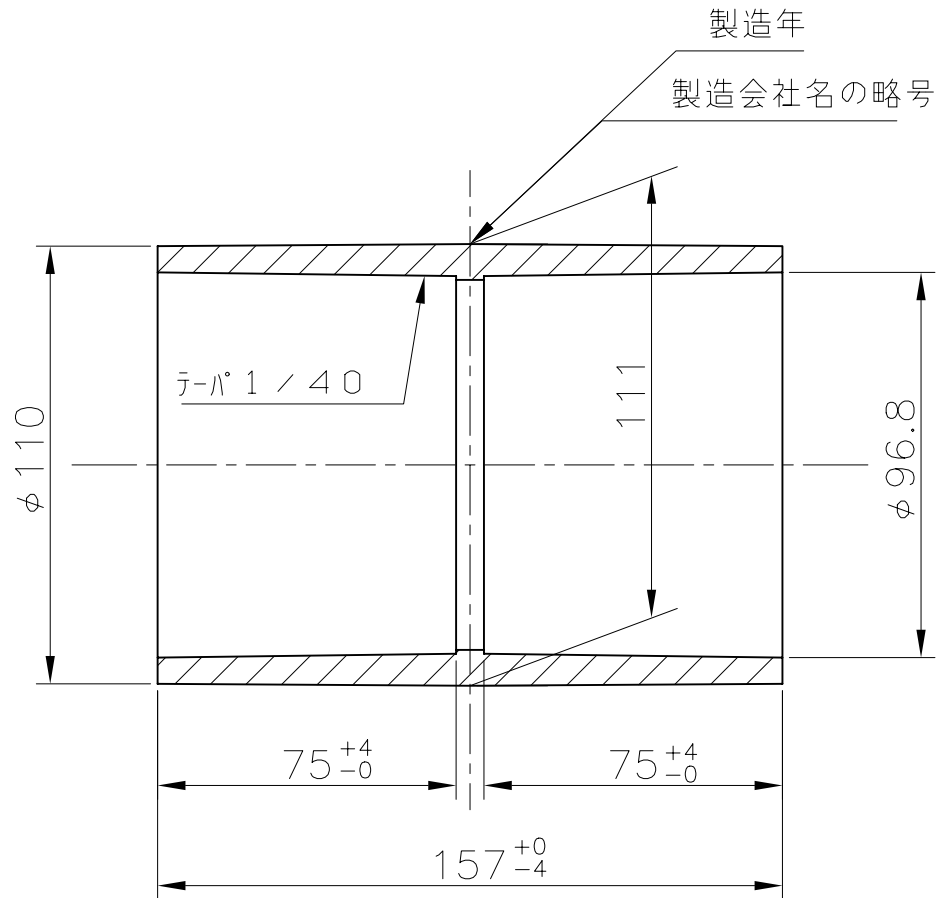
A-A断面
